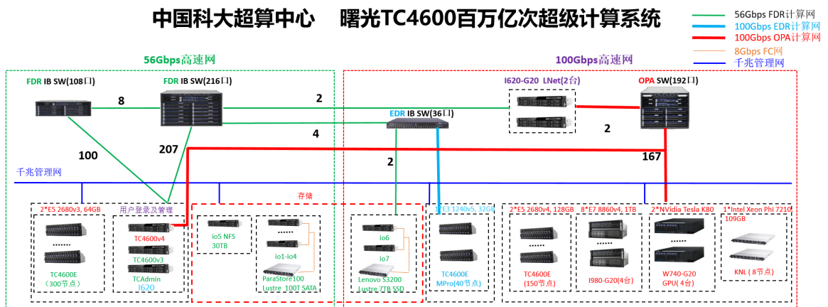
图 2: 曙光TC4600百万亿次超级计算系统拓扑
